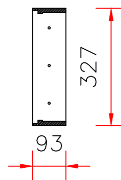
Bottomframe
